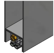
MONTAGE COMPLET : COUPER POUR FAIRE RENTRER DANS LA LARGEUR DE LA PORTE MOINS 1/16"
